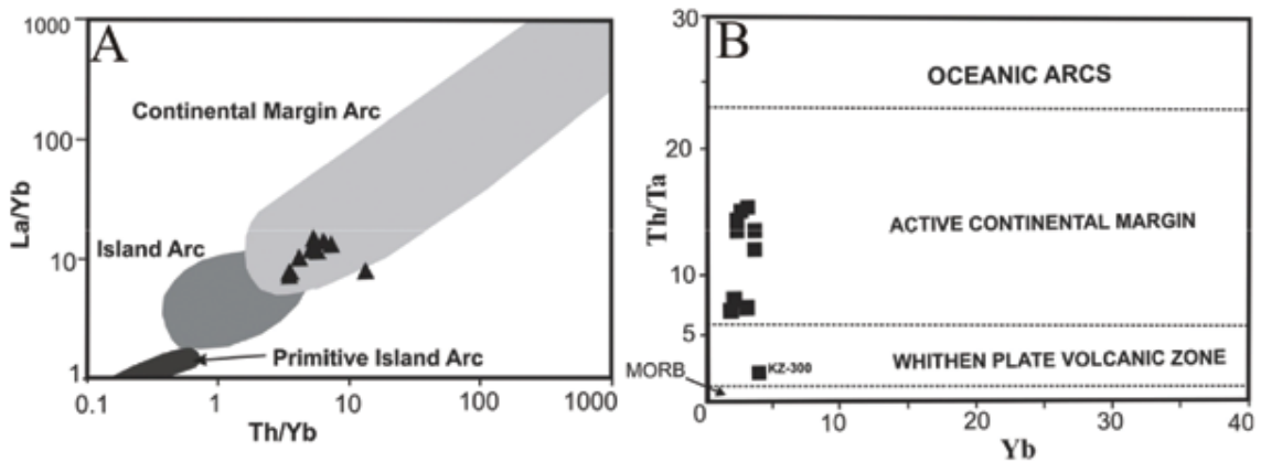
شکل ۱۱. نمودار Th/Yb در برابر La/Yb کمان حاشیه قاره (Condi, 1989). (B) نمودار Th/Ta در برابر Yb در برابر Yb (Gorton and Schandl, 2000)
