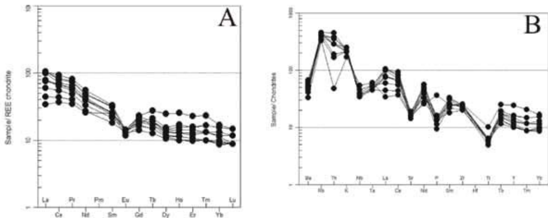
شکل ۹. تغییرات فراوانی عناصر نادر خاکی (REE) نرمالیز شده نسبت به کندریت (Sun and Mcdonough, 1989)، (B) تغییرات فراوانی عناصر فرعی و نادر خاکی نرمالیز شده نسبت به کندریت (Thompson, 1982)
