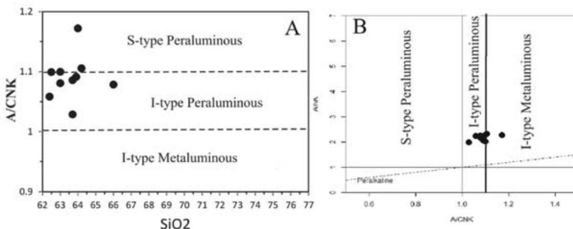
شکل ۷. نمودار تفکیک گرانیت‌ها بر اساس SiO_2 در برابر KNC/A (Chappell et al., 2012). (A) نمودار تفکیک گرانیت‌ها بر اساس شاخص اشباع از آلومینیم (Maniar and Piccoli, 1989). (B) نمودار تفکیک گرانیت‌ها بر اساس
