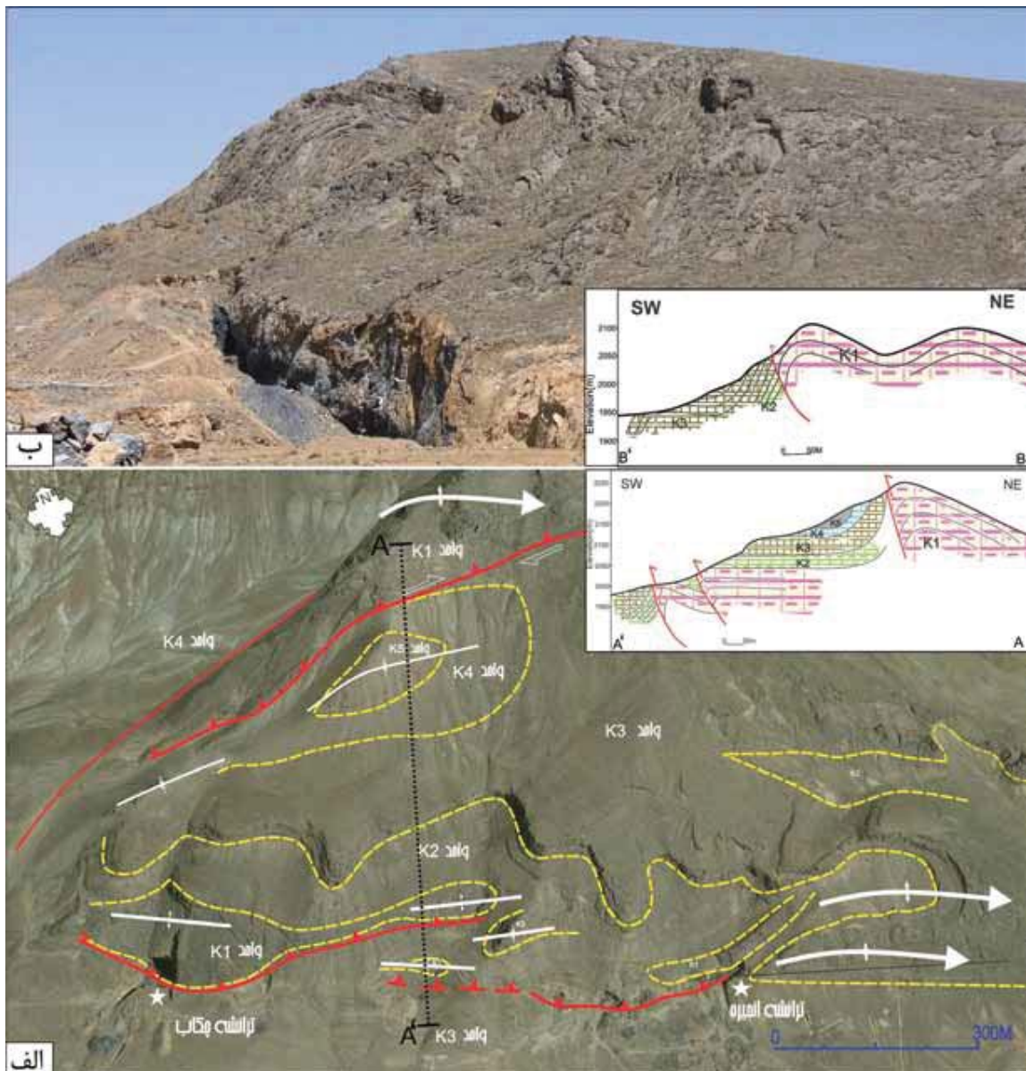
شکل ۲. الف) طاقدیس جنوب و جین بالا به همراه برش زمین‌شناسی B-B'. مطالعه نمونه در داخل ترانسه در مرز بین واحد K 1 و K 2 صورت گرفته است. جهت دید به سمت شمال باختر (ب) نمای کلی از واحدهای معدن انجیره - چکاب بر روی تصویر ماهواره‌ای (برگرفته از نرم افزار Google Earth) به همراه برش زمین‌شناسی A-A'
