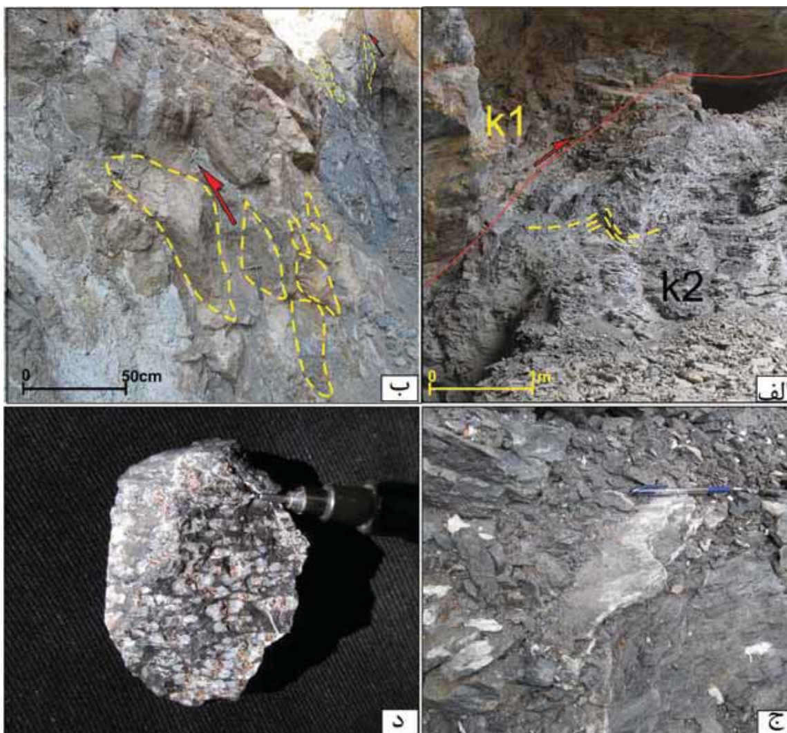
شکل ۳. نشانه‌های برشی برای حرکت معکوس به سمت جنوب باختر در پهنه برشی الف) ریزچین‌های موجود در پهنه برشی که در ترانشه‌های معادن وجین بالا و انجیره - چکاب دیده می‌شوند. این ریزچین‌ها هم روند با چین خوردگی اصلی بوده و با تمایل سطح محوری به سمت جنوب باختر قرار دارند. واحد K_1 در ترانشه‌ها با شیب به سمت شمال‌خاور، یال برگشته طاق‌دیس می‌باشند. ب) حالت‌های لنزی شکل از قطعات آهکی- شیلی در داخل ترانشه‌ها که حرکت معکوس به سمت جنوب باختر را نشان می‌دهند. ج) سطح گسل با رشته‌های کلسیتی. د) نمونه دستی از حاشیه کرنش موجود در اسفالریت‌ها
