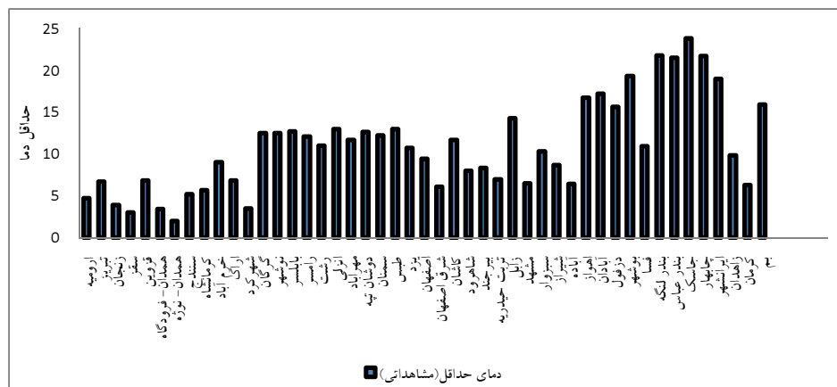
شکل ۲. میانگین دمای حداقل در ایستگاه‌های مورد مطالعه (۱۹۸۲-۲۰۱۲).
