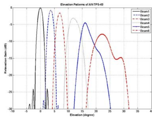
شکل ۷: پترنهای تشعشعی ارتفاع آنتن AN/TPS-۴۳ حاصل از نرم‌افزار پیشنهادی
