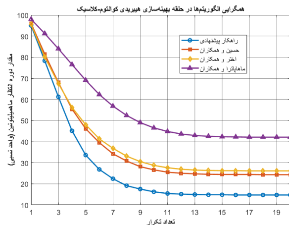
شکل ۷. نمودار همگرایی حلقه بهینه‌سازی مختلط کوانتومی -
