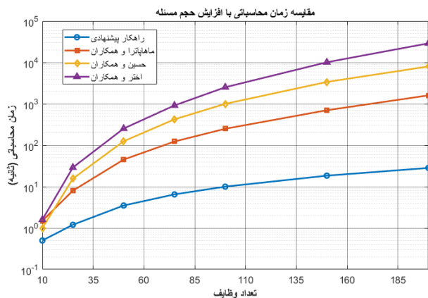
شکل ۳. مقایسه زمان محاسباتی با افزایش حجم مسئله (تعداد وظایف)
