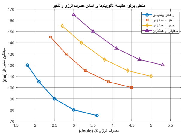
شکل ۵. مقایسه عملکرد الگوریتم‌ها در بهینه‌سازی چندهدفه تأخیر و مصرف انرژی
