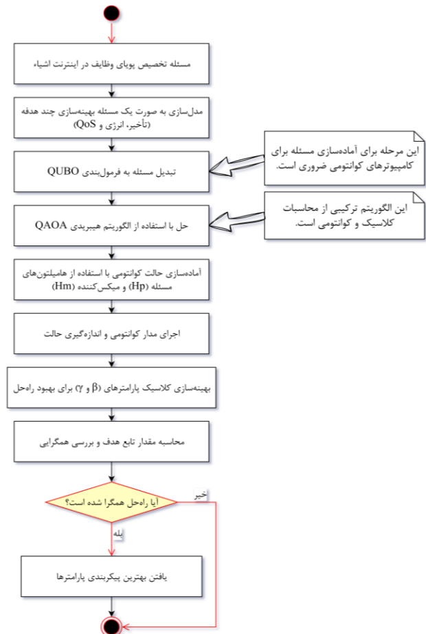
شکل ۲. روندنمای کلی رویکرد مختلط کوانتومی-سنتی برای حل مسئله تخصیص وظایف پویا در IoT
