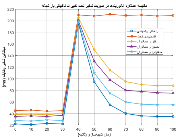
شکل ۶. مقایسه عملکرد پویایی سیستم در مدیریت تأخیر وظایف تحت تغییرات ناگهانی بار شبکه
