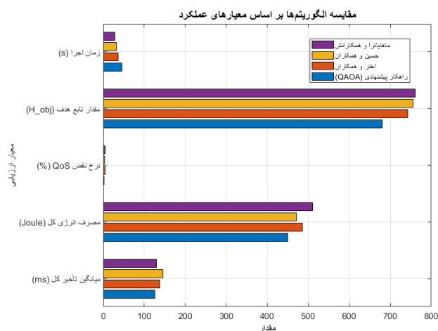
شکل ۴. تحلیل مقایسه‌ای عملکرد الگوریتم‌های بهینه‌سازی برای تخصیص وظایف
