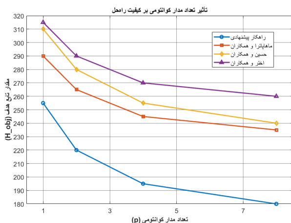
شکل ۸. تأثیر عمق مدار کوانتومی ( p ) بر کیفیت راه حل ( H_{obj} )
