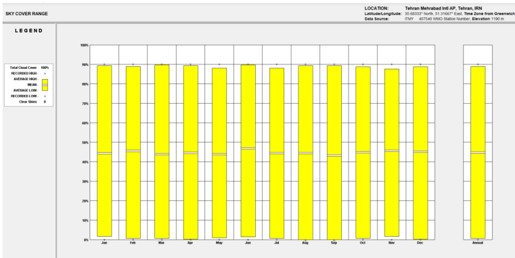
تصویر ۴- نمودار وضعیت پوشش آسمان ابری در شهر تهران در مقایسه با شرایط آسایش حرارتی در استاندارد اشری، استخراج شده از نرم‌افزار مشاور اقلیمی برحسب درصد
