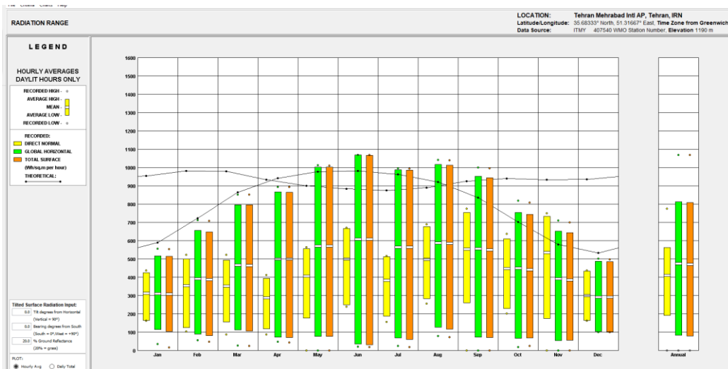
تصویر ۲- نمودار نوسان ساعتی تابش مستقیم و افقی در شهر تهران در مقایسه با شرایط آسایش حرارتی در استاندارد اشری، استخراج‌شده از نرم‌افزار مشاور اقلیمی (wh/sq.m per hour)
