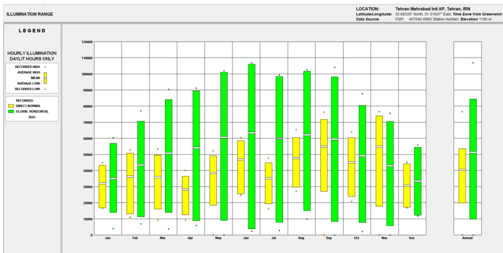
تصویر ۳- نمودار نوسان ساعتی روشنایی نور طبیعی در شهر تهران در مقایسه با شرایط آسایش حرارتی در استاندارد اشری، استخراج‌شده از نرم‌افزار مشاور اقلیمی برحسب لوکس
