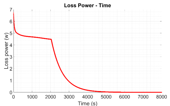
شکل ۹: تلفات اهمی باتری ناشی از شارژ با شیوه جریان ثابت-ولتاژ ثابت.
