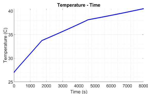
شکل ۱۳: تغییرات دمای باتری با شیوه جریان ثابت چندمرحله‌ای (شبیه‌سازی دوم).
