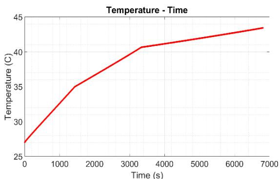
شکل ۱۶: تغییرات دمای باتری در روش شارژ سریع چندمرحله‌ای (شبیه‌سازی سوم).
