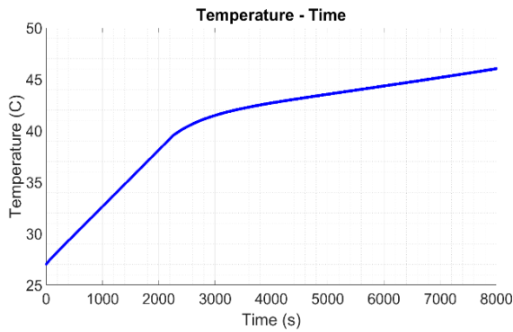
شکل ۱۰: تغییرات دمای باتری در زمان شارژ با شیوه جریان ثابت-ولتاژ ثابت.
