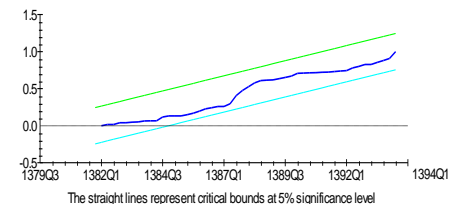
نمودار ۲- آزمون ثبات ساختاری CUSUMQ
