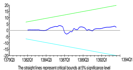
نمودار ۱- آزمون ثبات ساختاری CUSUM
