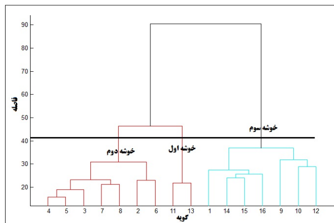
شکل ۴: دندروگرام حاصل از تحلیل خوشه‌ای برای گویه‌ها
