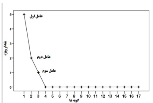
شکل ۲: نمودار سنگ‌ریزه برای مشخص کردن تعداد عامل‌ها
