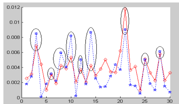
شکل ۴- مقادیر وزن مولفه‌های گاوسی (خطوط توپر) و توالی ۲ تایی مولفه‌های گاوسی (خطوط نقطه‌چین) برای زبان آلمانی
