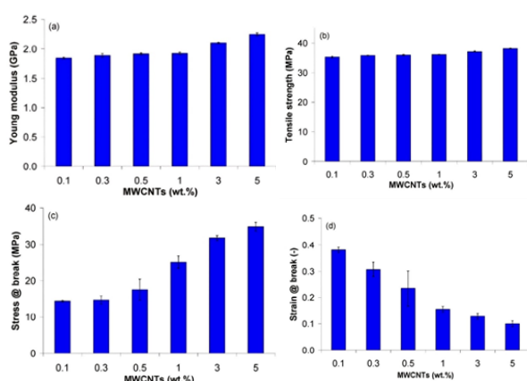
شکل ۳ خواص مکانیکی نانوکامپوزیت‌های PP/MWCNT: (a) مدول یانگ، (b) استحکام کششی، (c) تنش در نقطه شکست (d) کرنش در نقطه شکست در سرعت کشش ۱۰۰ میلی‌متر بر دقیقه [۲۱].
