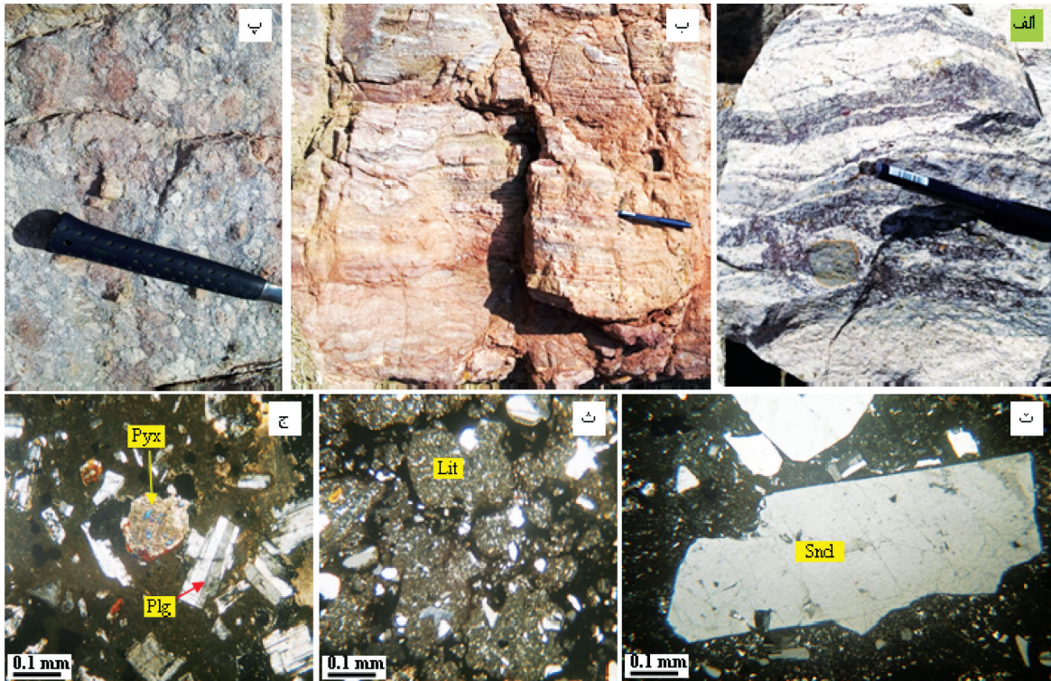
شکل ۳. الف) نمونه دستی از واحد ریولیتی با بافت جریان‌ی، ب) تصویر رخنمونی از واحد توفی با لایه‌بندی ظریف، پ) رخنمونی از واحد آذرآواری لیتیک توف، ت) تصویر میکروسکوپی از واحد ریولیتی که دارای کانی سانیدین (Snd) است (XPL)، ث) تصویر میکروسکوپی از واحد توفی با فراوانی قطعات لیتیک (Lit) (XPL)، ج) تصویر میکروسکوپی از واحد آندزیت بازالتی متشکل از پلاژیوکلاز (Plg) و پیروکسن (Pyx) (XPL)
