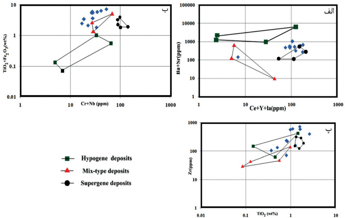
شکل ۸. الف) نمودار Ba+Sr در مقابل Ca+Y+La، بیشتر نمونه‌ها در محدوده سیالات سوپرژن قرار می‌گیرند، ب) نمودار TiO_2+Fe_2O_3 در مقابل Cr+Nb (Dill et al, 1997) در مقابل Zr در مقابل TiO_2 (Maiza et al., 2003) جهت تعیین منشأ محلول دگرسان
