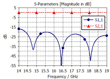
شکل ۷: افت بازگشتی ( |S_{11}| ) و تلف عبوری ( |S_{21}| ) شبیه‌سازی شده موجبر RGW.
