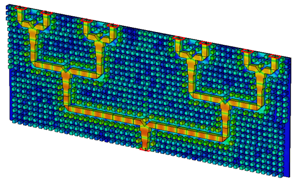
شکل ۱۴: حرکت موج در مقسم توان ۱۸ با استفاده از ساختار دودویی RGW (فرکانس ۱۶.۵ GHz).
