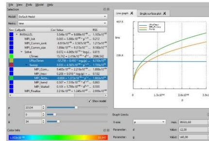
شکل ۷ نمای خروجی مدل Extra-P [۳۹]
