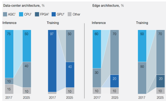
شکل ۱۱. روند تغییر سهم فناوری‌های سخت افزاری در تعداد موارد استفاده در کاربردهای یادگیری عمیق [۵۱]
