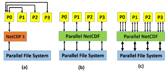
شکل ۴ مقایسه‌ی دسترسی به فایل در حالت NetCDF متوالی و Parallel NetCDF [۳۶]
