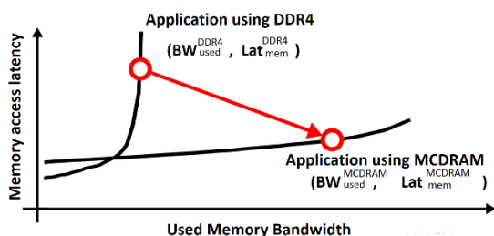
شکل ۶ تخمین PROFET برای سیستم حافظه‌ی هدف [۳۸]
