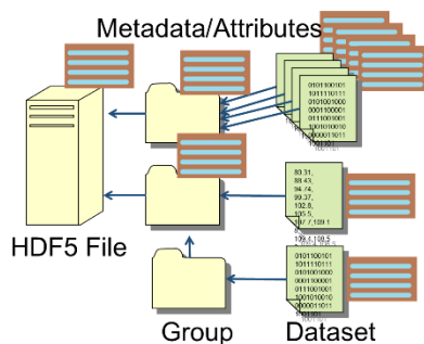
شکل ۳ ساختار فرمت فایل HDF5 [۳۵]
