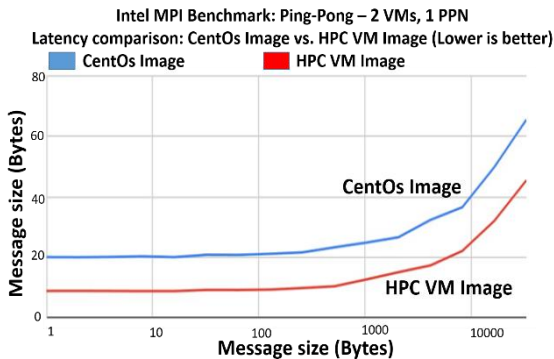
شکل ۱۴. کاهش تاخیر MPI با استفاده از HPC VM Images [۵۵]
