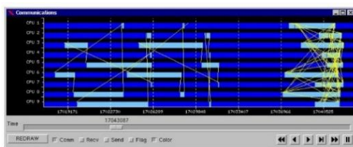
شکل ۹ نمای خروجی مدل Paraver [۴۱]
