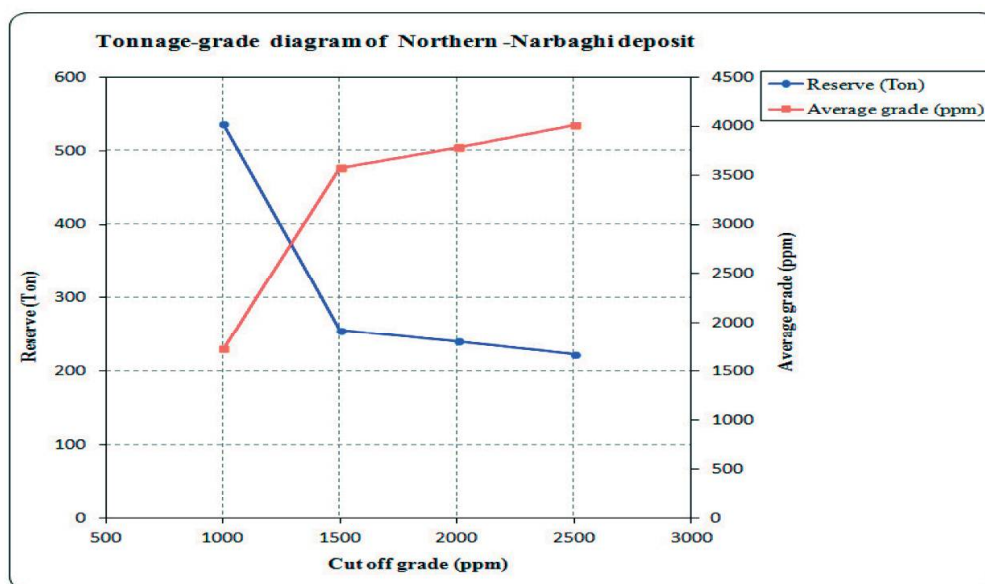
شکل ۷. نمودار عیار-تناژ کانسار مس نارباغی شمالی با روش لاگ کریجینگ معمولی با استفاده از SGeMS
