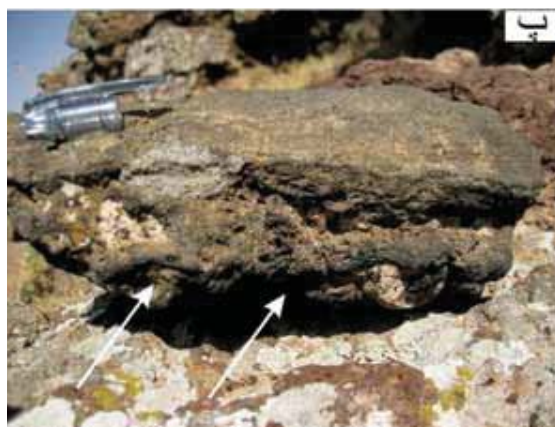
شکل ۴. الف) دهانه به شکل مخروط سیندر و یا مخروط اسکوری، ب) گدازه آآ در بخش بالایی مخروط سیندر خاتون باغ، پ) دوک با آثار تاپاله‌گاوی در سطح زیر آن در دهانه مخروط سیندر
