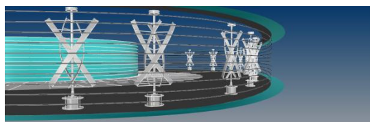
شکل ۱۲- توربین و نحوه عملکرد آن در برج رودخانه پرل (پیتترست برج رودخانه پرل).
