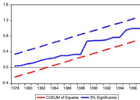
نمودار (۲) - آزمون پایداری ضرایب CUSUMQ
