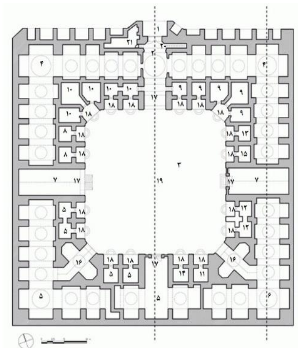
شکل ۲. کاروانسرای شاه عباسی در کاربری مدرسه بزرگان دوره قاجاریه (منبع: میراث‌فرهنگی)
