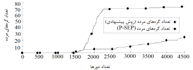
شکل ۱۹: مقایسه تعداد گره‌های مرده بین پروتکل پیشنهادی و پروتکل P-SEP برای شبکه با اندازه ۱۰۰، \alpha = 3 ، m = 0.3 و تعداد دور ۴۵۰۰.
