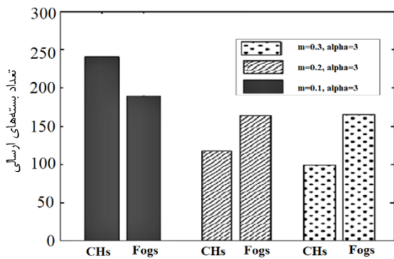
شکل ۷: تعداد بسته‌های ارسالی به گره‌های مه در پروتکل پیشنهادی برای شبکه با اندازه ۵۰۰، \alpha = 3 ، و مقادیر مختلف m و تعداد دور ۴۵۰۰.
