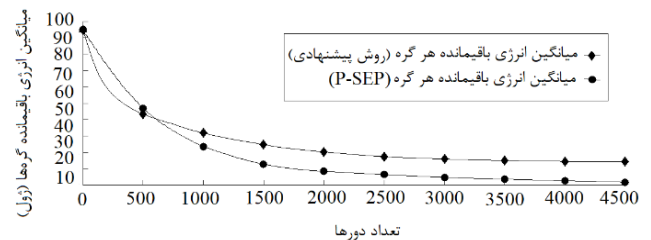
شکل ۲۰: مقایسه میانگین انرژی باقیمانده بین پروتکل پیشنهادی و پروتکل P-SEP برای شبکه با اندازه ۵۰۰، \alpha = 3 ، m = 0.3 و تعداد دور ۴۵۰۰.
