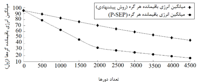
شکل ۲۱: مقایسه میانگین انرژی باقیمانده بین پروتکل پیشنهادی و پروتکل P-SEP برای شبکه با اندازه ۱۰۰، \alpha = 3 ، m = 0.3 و تعداد دور ۴۵۰۰.
