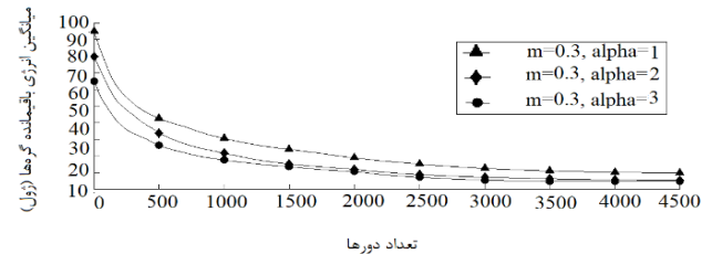
شکل ۵: میانگین انرژی باقیمانده برای هر گره در الگوریتم پیشنهادی برای اندازه شبکه ۵۰۰، m = 0.3 و مقادیر مختلف تعداد دور ۴۵۰۰.
