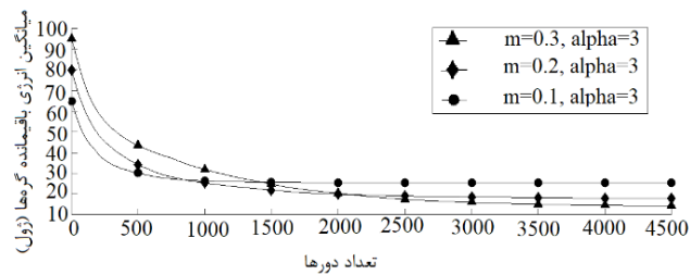
شکل ۳: میانگین انرژی باقیمانده برای هر گره در الگوریتم پیشنهادی برای اندازه شبکه ۵۰۰، \alpha = 3 ، مقادیر مختلف m و تعداد دور ۴۵۰۰.
