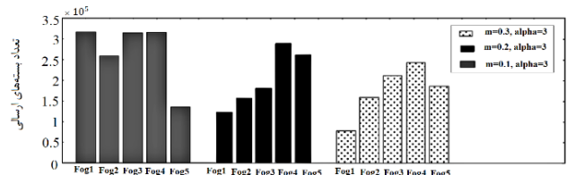
شکل ۶: تعداد بسته‌های انتقالی به گره‌های مه در پروتکل پیشنهادی برای شبکه با اندازه ۵۰۰، \alpha = 3 ، و مقادیر مختلف m و تعداد دور ۴۵۰۰.
