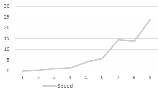
شکل ۲۳: زمان اجرای الگوریتم PADC در چارچوب MapReduce بر اساس تعداد ورودی‌ها در مجموعه داده ۲M - Power consumption با ۴ گره اجرایی.
