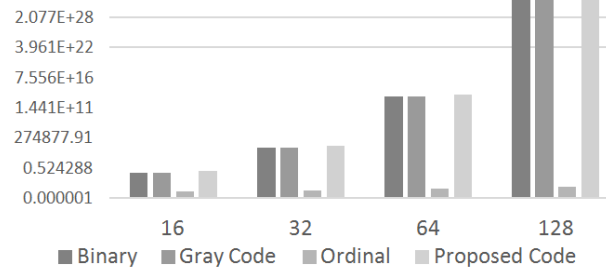
شکل ۲۸: میزان حافظه مصرفی کدگذاری ها در مجموعه داده تولیدی تصادفی.
