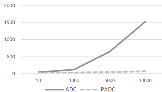
شکل ۲۹: مقایسه زمان اجرای دو الگوریتم (۱۶ Thread) ADC و PADC در مجموعه داده ۱۰k - No-show.
