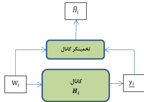
شکل ۲: تخمینگر کانال.
