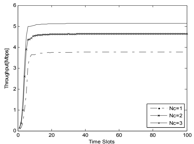
شکل ۵: اثر تعداد سلول های هماهنگ بر گذردهی سلول.
