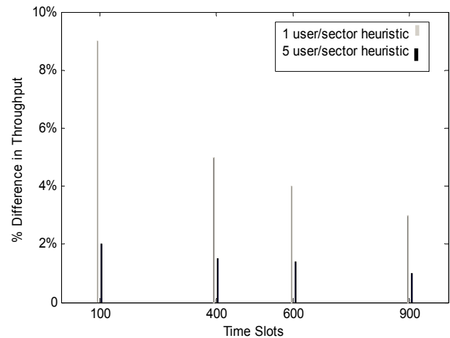
شکل ۴: درصد اختلاف گذردهی سلول در زمان بندی ابتکاری نسبت به زمان بندی بهینه.
