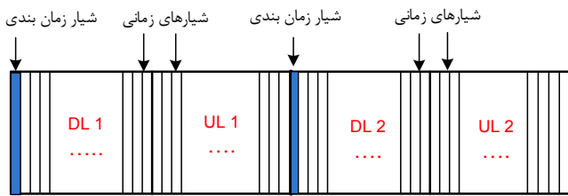
شکل ۲: قاب‌ها و شمارهای زمانی در مسیر بالاسو و پایین‌سو.
