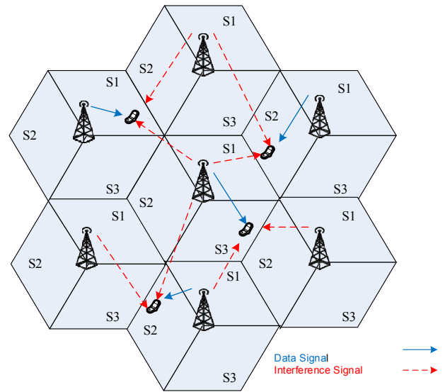
شکل ۱: مدل سیستم زمان‌بندی هماهنگ عادلانه با قطاع‌بندی سلول.
