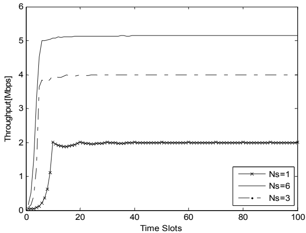
شکل ۳: اثر قطاع بندی سلول بر گذردهی سلول.
