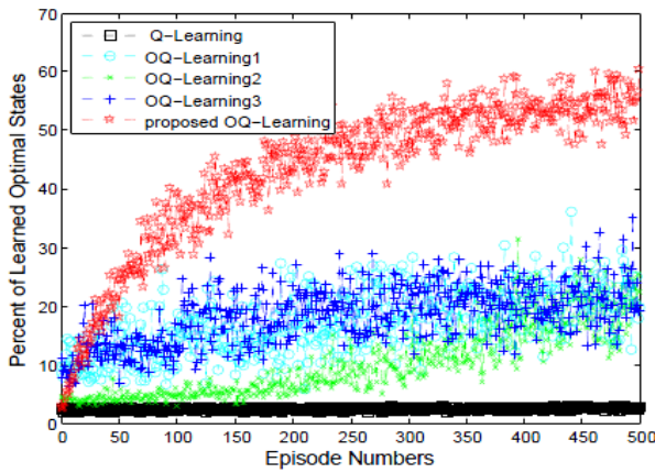
شکل ۶: میانگین درصد بهینه به تعداد دوره‌ها در محیط ۱۰×۱۰ با پارامترهای \alpha=0.3 و \gamma=0.9 .
