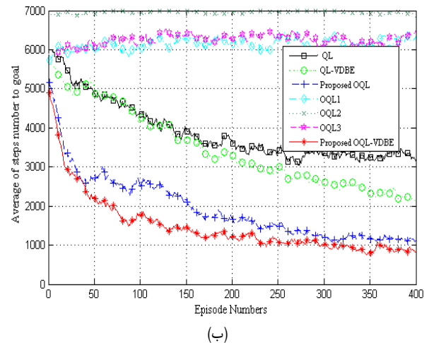
شکل ۱۱: میانگین تعداد گام‌ها به تعداد دوره‌ها با \alpha = 0.1 و \gamma = 0.7 ، (الف) محیط 24 \times 24 و (ب) محیط 48 \times 48 .
