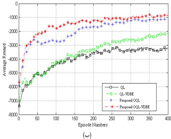
شکل ۱۰: میانگین تعداد پاداش به تعداد دوره‌ها با \alpha = 0.1 و \gamma = 0.7 ، (الف) محیط 24 \times 24 و (ب) محیط 48 \times 48 .
