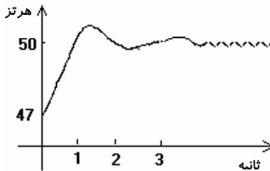
شکل ۱۱: تغییر خروجی سرعت دیزل ژنراتور از زمان آغاز کار سنکرونایزر.
