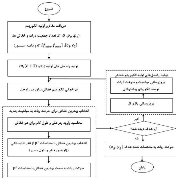
شکل ۲. فلوچارت خلاصه مراحل روش پیشنهادی برای
