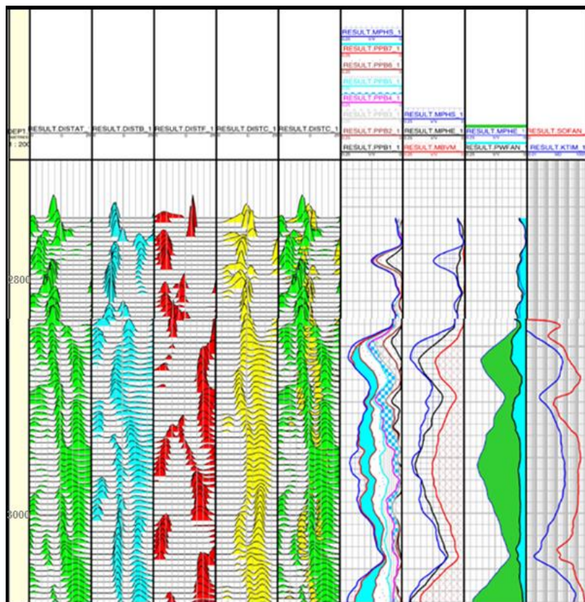
شکل ۸) زمان آرمیدگی T_2 در حفرات مختلف چاه شماره ۱۹ همراه با سیالات مختلف
