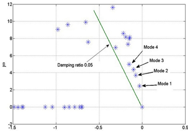
شکل ۴: مکان مدهای سیستم قبل از بهینه‌سازی و نصب ادوات FACTS.
