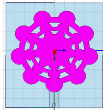
شکل ۷: ساختار آنتن پیشنهادی در تکرار دوم.
