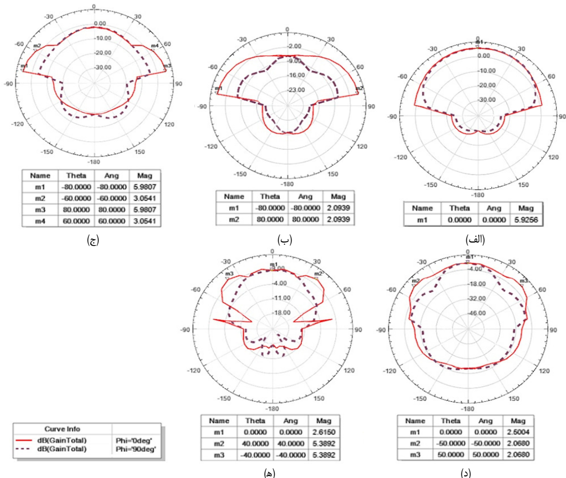
شکل ۱۶: پترن تشعشی آنتن و بهره در فرکانس های تشدید، الف) ۱٫۹ GHz، ب) ۴٫۴ GHz، ج) ۵٫۶ GHz، د) ۷٫۸ GHz و ه) ۸٫۵ GHz خط پر \varphi = 0^\circ و خطچین \varphi = 90^\circ .
