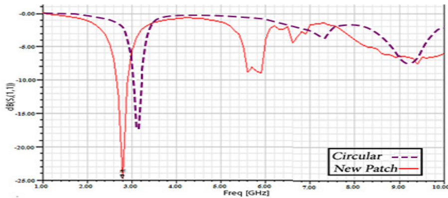
شکل ۳: نمودار شبیه‌سازی S_{11} برای آنتن با پیچ دایروی ساده و پیچ تغییر یافته در شکل ۳.
