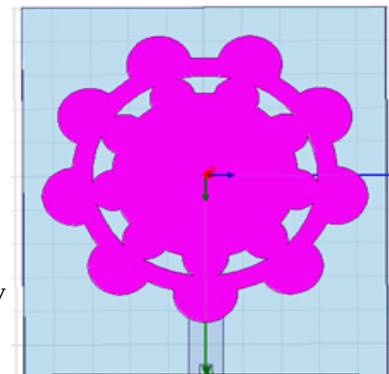
شکل ۵: ساختار آنتن پیشنهادی در تکرار اول.
