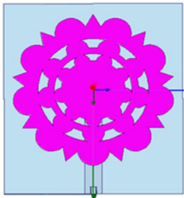
شکل ۹: آنتن فرکتال با افزایش طول الکتریکی توسط مثلث در لبه.
