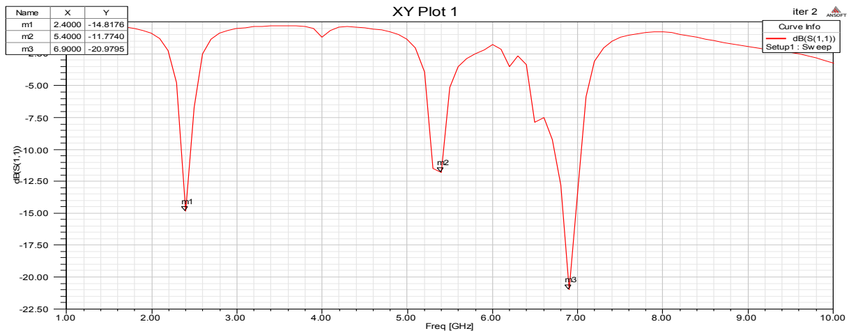
شکل ۴: نتایج شبیه‌سازی S_{11} آنتن با تکرار اول ساختار شکل ۵.
