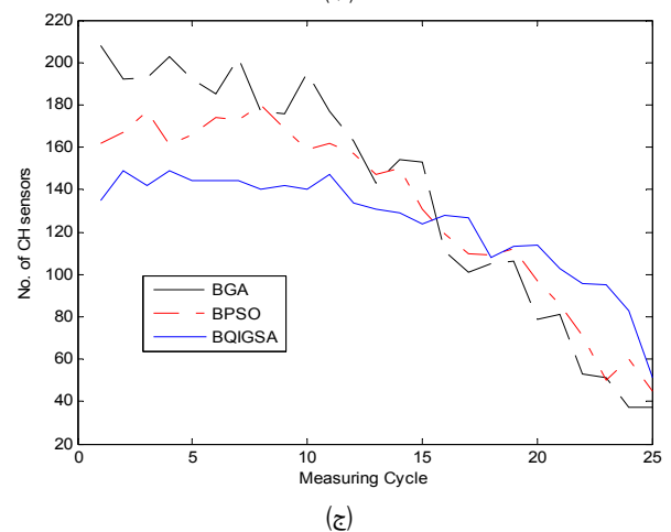
شکل ۶: ارزیابی عملکرد سه الگوریتم BGA، BPSO و IBGSA در ۲۵ دوره اندازه‌گیری، (الف) مقدار تابع هدف، (ب) پارامتر انرژی عملیاتی، (ج) تعداد حسگرهای سرگروه، (د) تعداد حسگرهای منظم با محدوده حسگری بلند، (ه) تعداد حسگرهای با محدوده حسگری کوتاه و (و) پارامتر انرژی ارتباطی.
