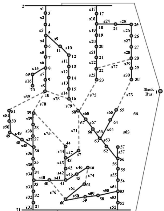
شکل ۸: دیاگرام شبکه توزیع ۷۰ شینه.
