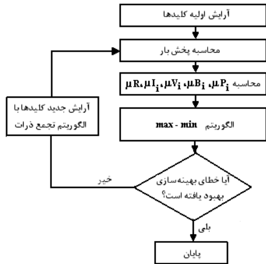
شکل ۶: دیاگرام بلوکی الگوریتم پیشنهادشده.
